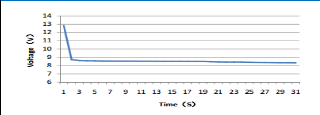
Cold Cranking Test Graph (-18°C, 780CCA)
