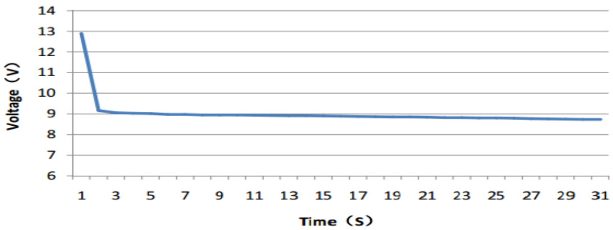
Cold Cranking Test Graph (-18°C, 330CCA)
